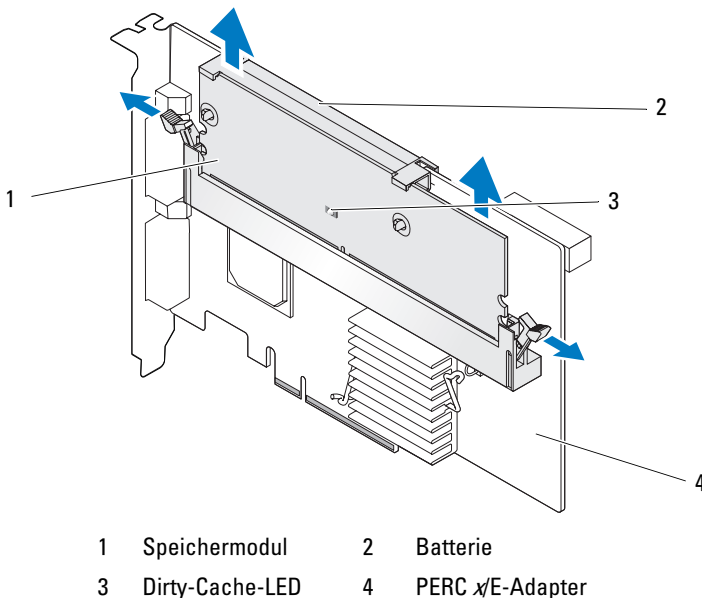
Abbildung 1. Position der Dirty-Cache-LED am PERC x/E-Adapter
